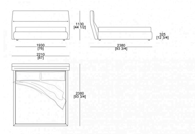
Letto (materasso L. 1930 x P. 2020 mm)
